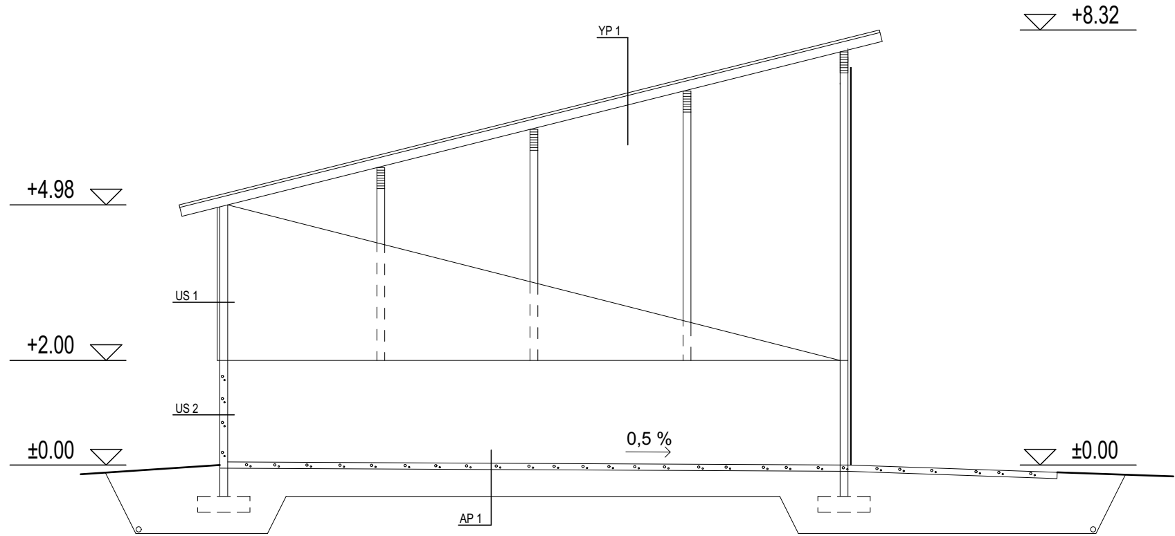
LEIKKAUS A-A
