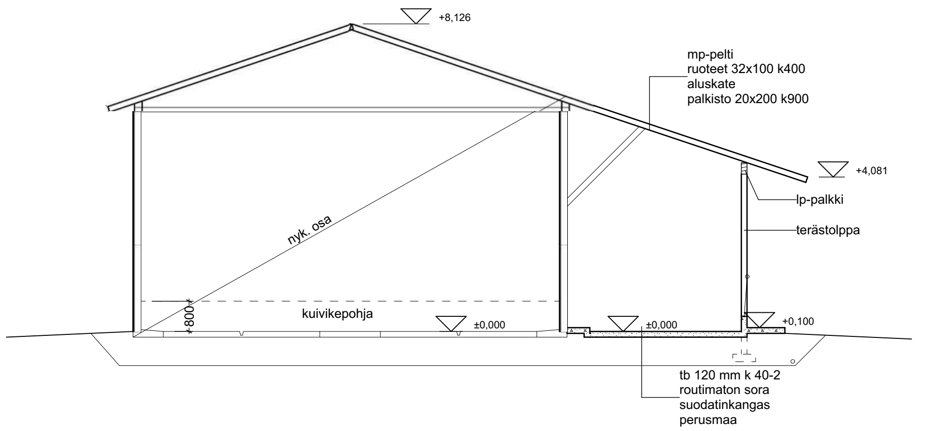
LEIKKAUS A-A
